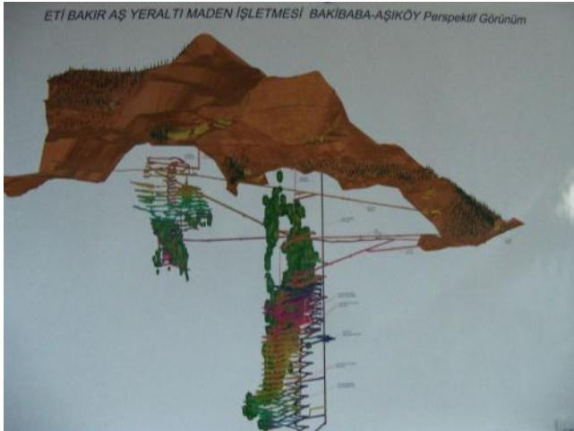
Küre Yeraltı Maden İşletmesi Perspektif Görünümü
